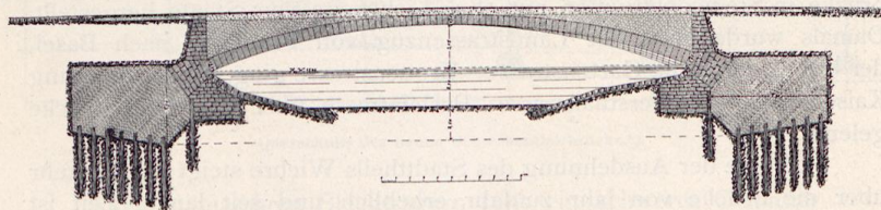
Längenschnitt des Entwurfs zur neuen Kaiserstrassenbrücke*).
