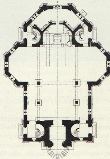
Grundriss der evangelischen Christus-Kirche.
