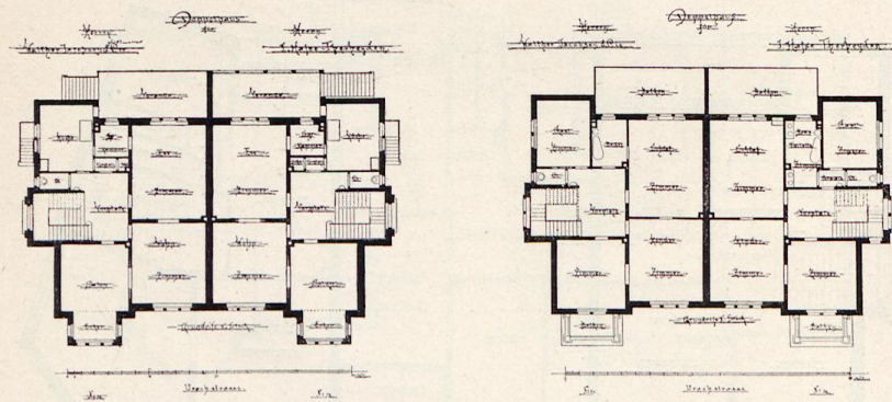
Doppelhaus J. Hasse-Therheyden und Fr. Jacobsen, Urachstrasse. Architekten: Walther, Jacobsen und Fr. Bauer.
