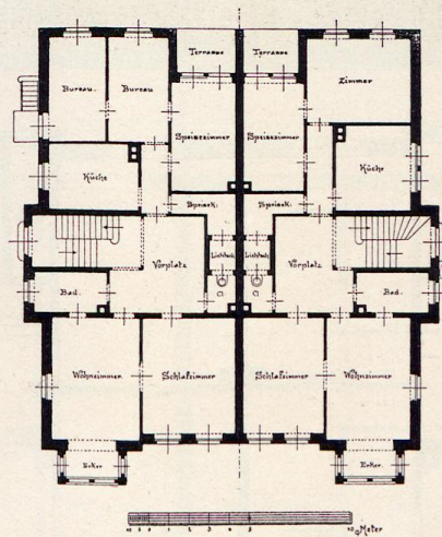
Doppelwohnhaus Uhlandstrasse No. 7 und 9. Eigentümer von No. 7: Jos. Mayer, Maurermeister. Eigentümer von No. 9: E. Brüttsch, Architect. Architect: E. Brüttsch. Baukosten (von Sockelunterkante bis Hauptgesimsoberkante gerechnet): 20 Mk. per cbm.
