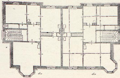
Doppelvilla Goethestrasse. — Eigenthümer von No. 10: Hofrath Rümelin, Baukosten 52,000 Mk. Eigenthümer von No. 12: Privat Ritgen, Baukosten 50,000 Mk. — Architect: W.Meess.
