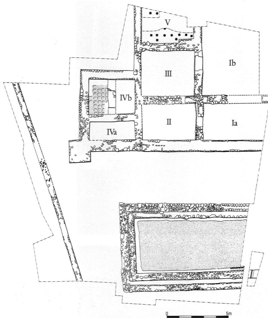
Abb. 2: Plan der beiden römischen Gebäude. Oben: Eckbereich des Wohngebäudes mit Badetrakt (IVb: Kaltwasserwanne, V: Hypocaustraum); unten: Bau mit großem, flachem Wasserbecken.
