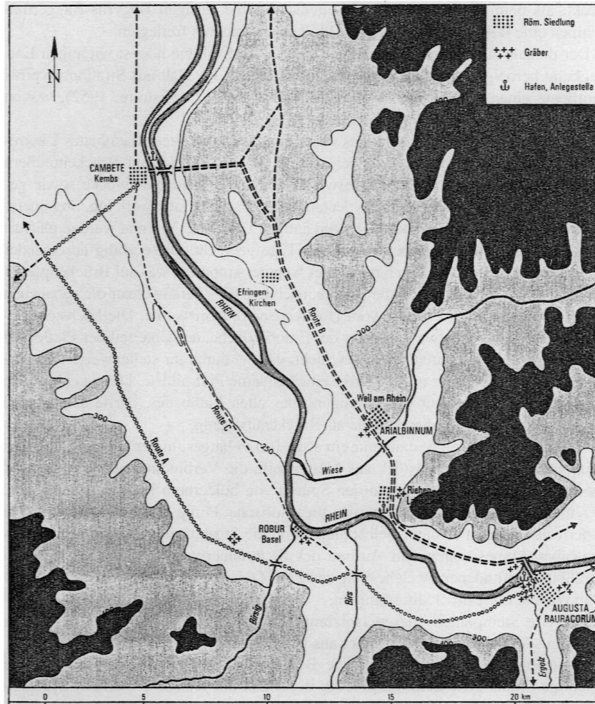
Abb.2: Das römische Straßennetz am Oberrhein mit der hypothetischen Brücke bei Kembs
