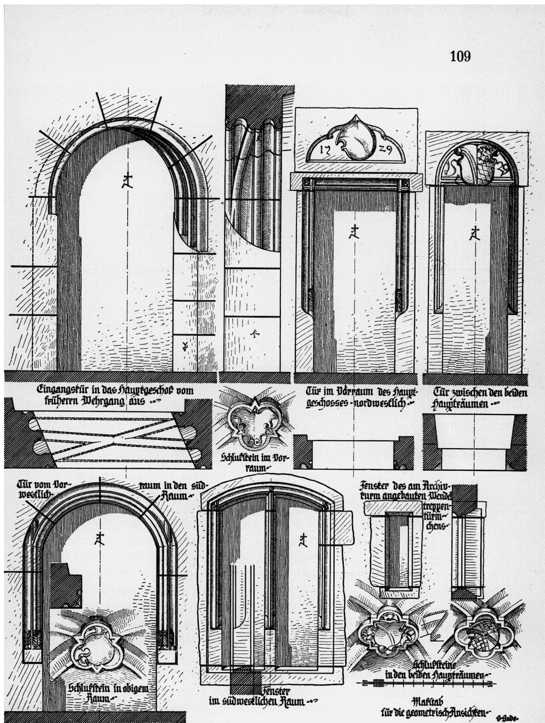
Abb. 14. Tür-, Fenster- und Gewölbefußsteindetails des Archivturms.
