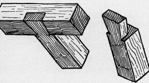
Abb. 3. Blatt mit Schwalbenschwanz.
