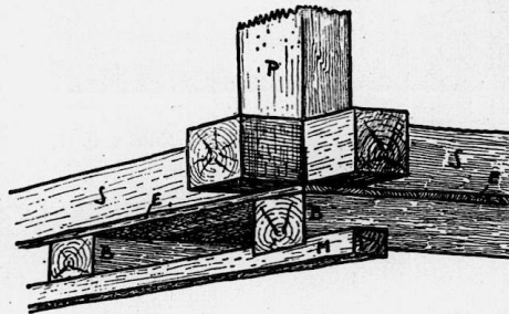
Abb. 38. Feffenbach, Haus Nr. 70, untere Hausecke.
