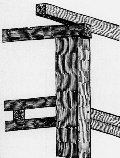
Abb. 39. Schutterwald, Haus Nr. 67, vordere Hausecke.
