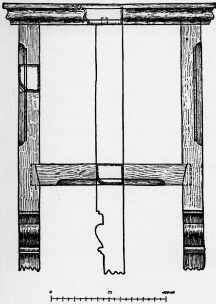
Abb. 36. Ohlsbach, Haus Nr. 125, Fenstereinzelleiten.
