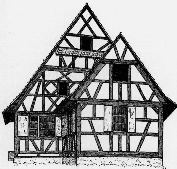
Abb. 61. Zell-Weierbach, Haus Nr. 93, aus dem Jahre 1763.
