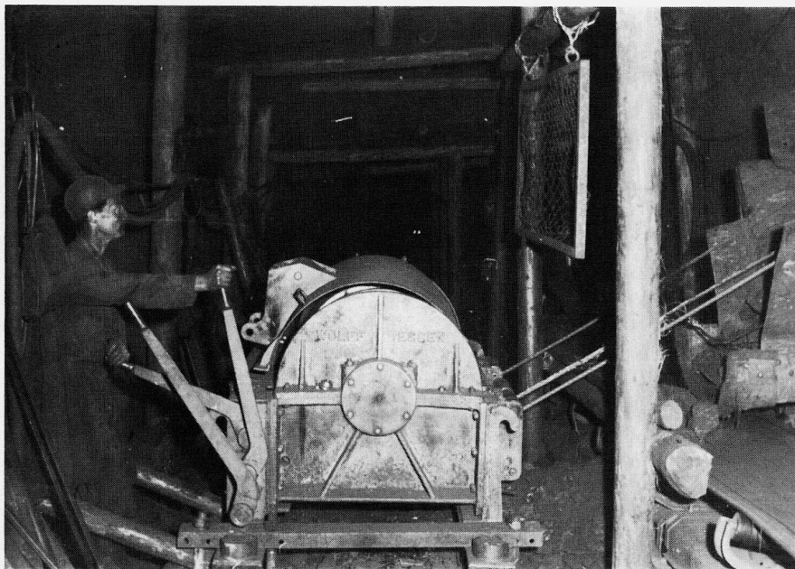
Stollen I: Schrapperhaspel in der Förderstrecke (1956)
