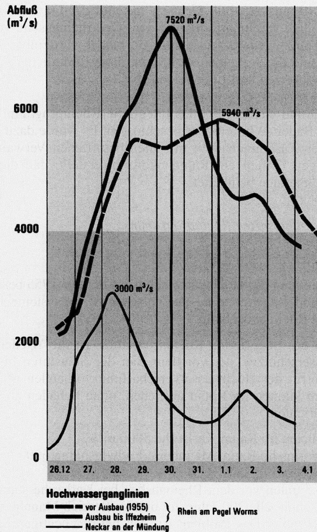
Abb. 2. Erhöhung der Hochwasserspitzen durch den Rheinausbau.
