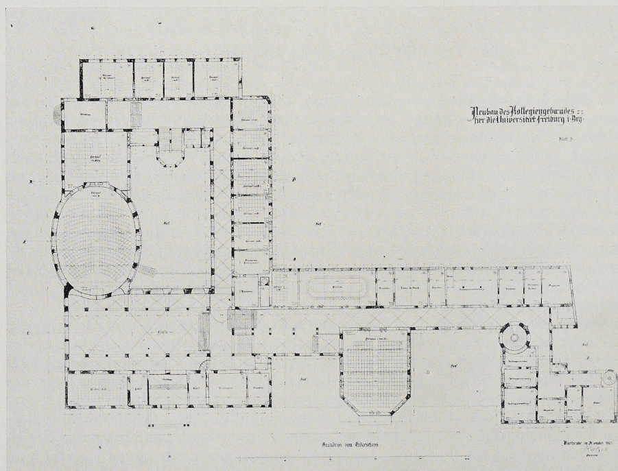
Abb. 7 Kollegiengebäude, Grundriß des Erdgeschosses
